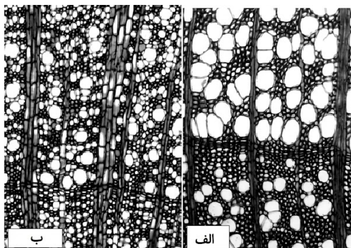
شکل ۲۵: ساختار چوب در سرشاخه‌های هم‌سن درخت Fagus sylvatica برداشت شده از شرایط نور بهینه (الف) و نور کمینه (ب). (بزرگنمایی تصاویر ۱۰۰ برابر).
