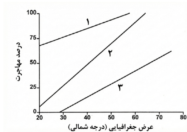
شکل ۲۹: درصد پرندگان مهاجر در هر عرض جغرافیایی
